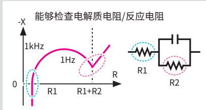
电池阻抗分析仪BT4560-60/化学阻抗分析仪IM3590
