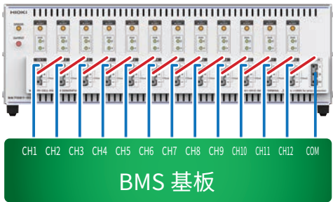
12 通道连接示例
