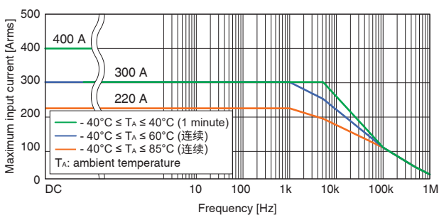
频率特性(典型特性)
