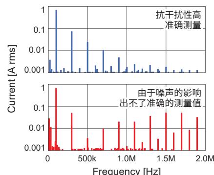
上: CT6904A CMRR 120 dB 以上 (100 Hz) 下: CMRR低的传感器
