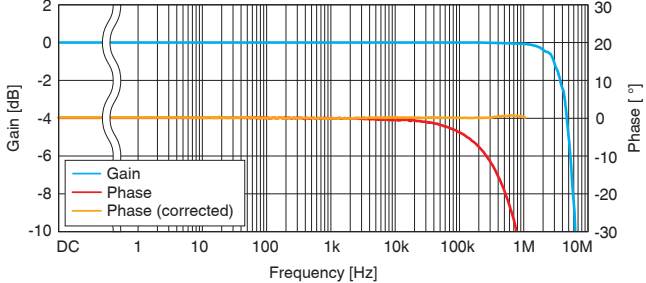
频率特性(典型特性)
