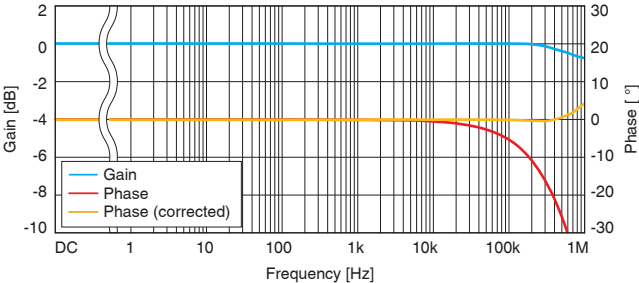
频率特性(典型特性)
